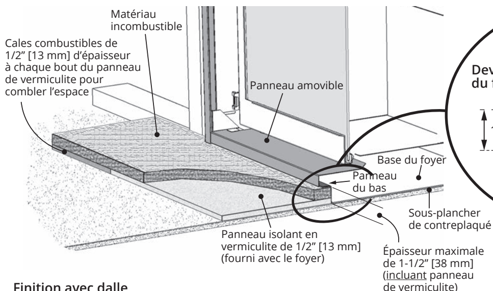
Finition avec dalle
