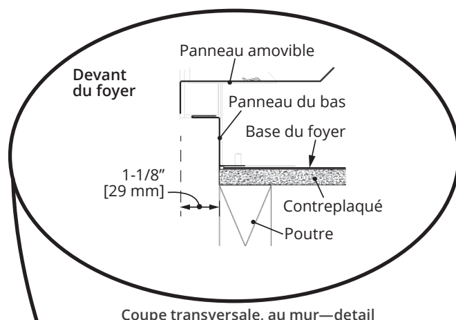
Coupe transversale, au mur—détail
