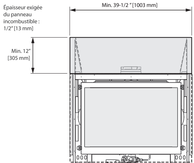
Dimensions minimales du panneau incombustible
