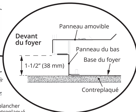
Coupe transversale, dalle—détail
