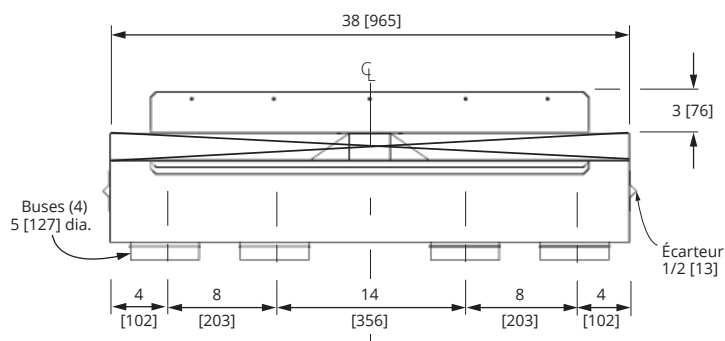
Vue avant
