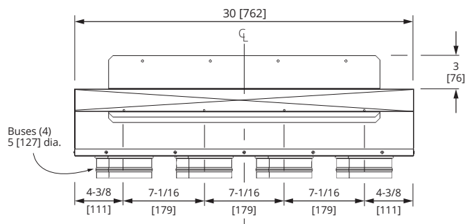
Vue avant
