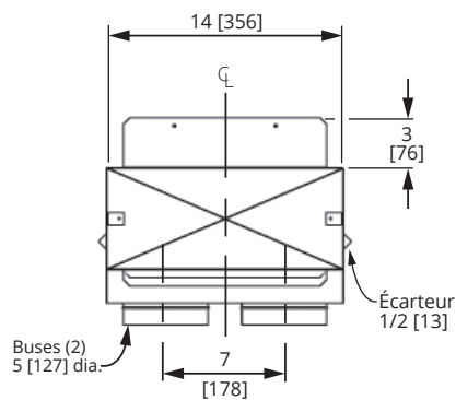
Vue avant
